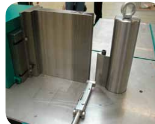
Prismaverlängerung Vee-block extension
