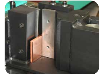
Schneidwerkzeug Shear tool
